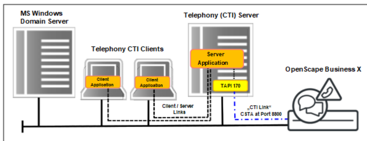
Abbildung 13: Serverbasierte TAPI-Applikation über TAPI 170 an OpenScape Business
